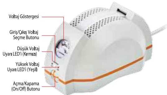
Ön Görünüş
